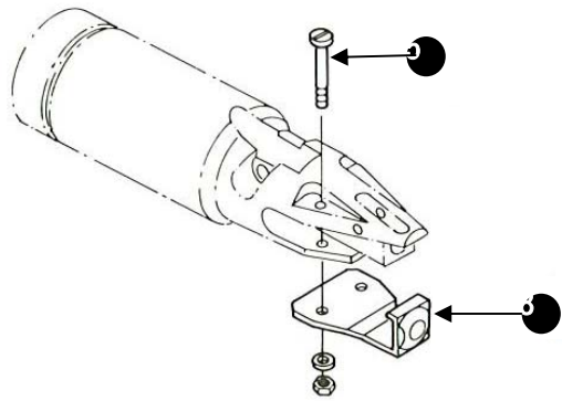
ガイド治具
