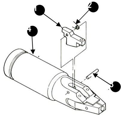
反転防止爪付型Yパイプ
